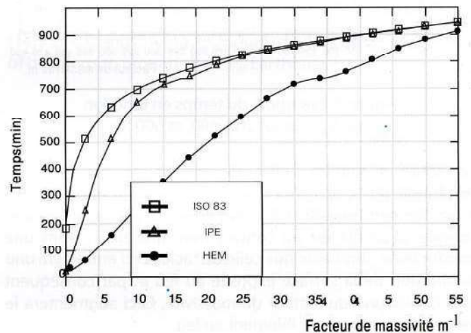
Figure 2: Évolution de la température de deux éléments non protégés
