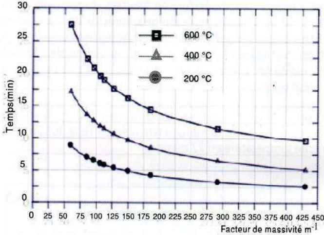
Figure 4: Evolution du temps en fonction de A_m/V pour 200, 400, et 600 °C
