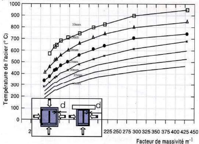
Figure 5: Température en fonction de A_m/V pour des aciers protégés après 1h 30mn d'incendie
