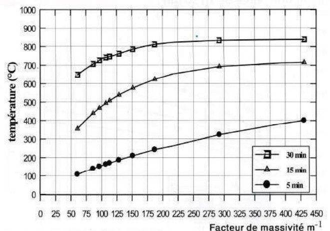
Figure 3: Evolution de la température en fonction de A_m/V pour 5, 15 et 30 min
