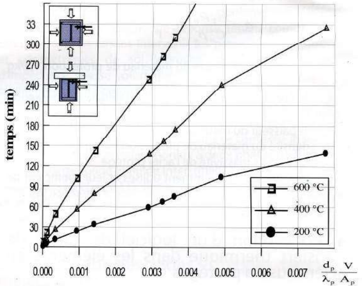
Figure 6: Temps de résistance en fonction du facteur ( d_p V/\lambda_p A_p )
