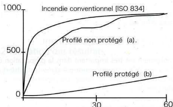
Figure 1 : Echauffement d'un profilé en acier en fonction du type de protection thermique
